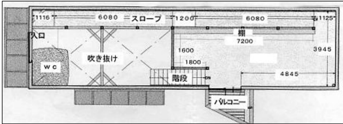
【平面図】
